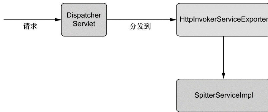
图15.8 HttpInvokerServiceExporter工作方式与Hessian和Burlap很相似，通过Spring MVC的DispatcherServlet接收请求，并将这些请求转换成对Spring bean的方法调用
