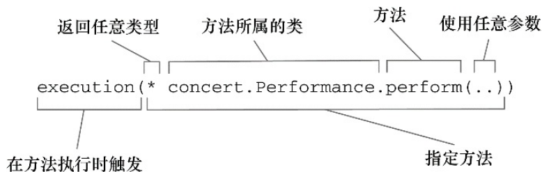
图4.4 使用AspectJ切点表达式来选择Performance的perform()方法
