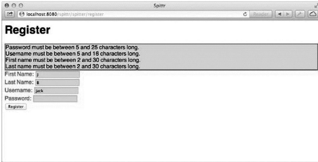
图6.3 显示校验错误，其中这些对用户友好的信息是从属性文件中获取到的
