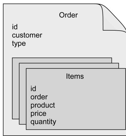
图12.1 文档展现了关联但非规范化的数据。 相关的概念(如订单中的条目)被嵌入到顶层的文档数据中
