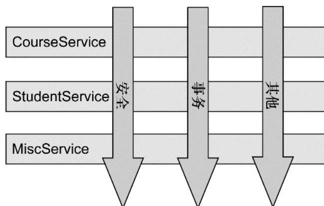
图4.1 切面实现了横切关注点(跨多个应用对象的逻辑)的模块化
