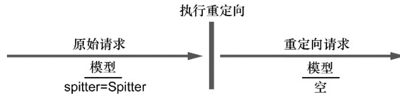
图7.1 模型的属性是以请求属性的形式存放在请求中的,在重定向后无法存活
