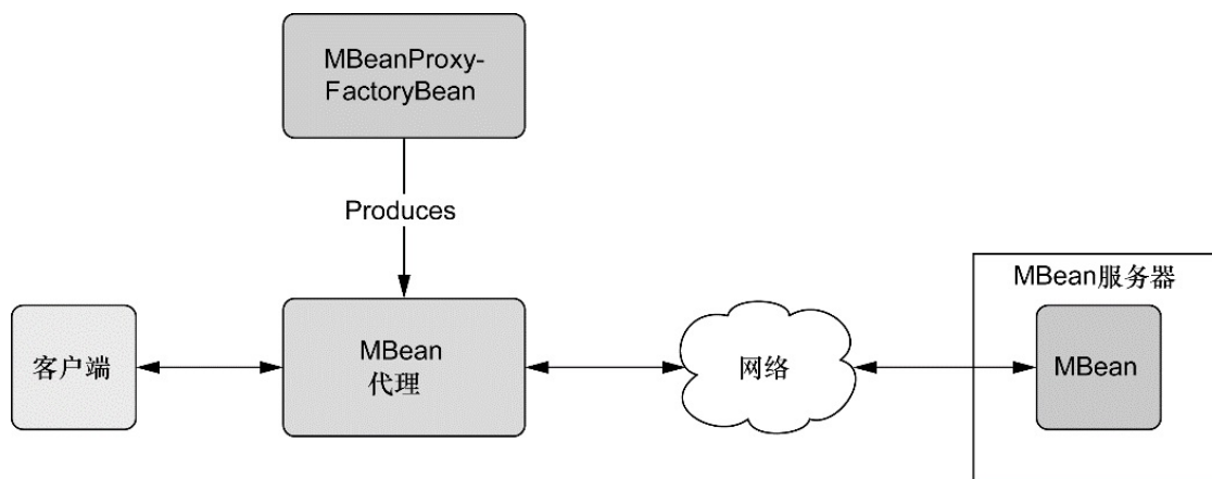
图20.4 MBeanProxyFactoryBean创建远程MBean的代理。客户端通过此代理与远程MBean进行交互，就像它是本地Bean一样
