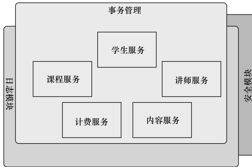
图1.3 利用AOP，系统范围内的关注点覆盖在它们所影响组件之上
